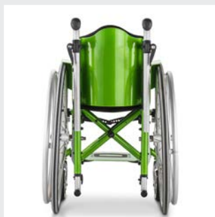
Coque de dossier anatomique en aluminium, amovible
